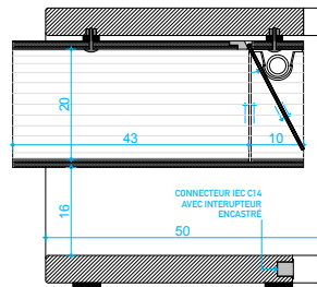
COUPE TRANSVERSALE
